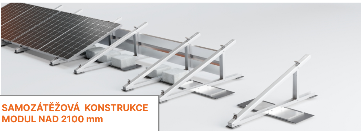
JIH 15/20° BIFACIAL NA SENDVIČOVÝ PANEL
