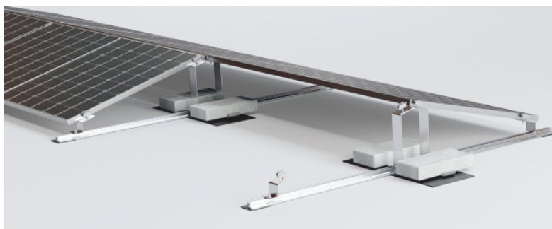
SAMOZÁTĚŽOVÁ KONSTRUKCE AERO VÝCHOD-ZÁPAD
