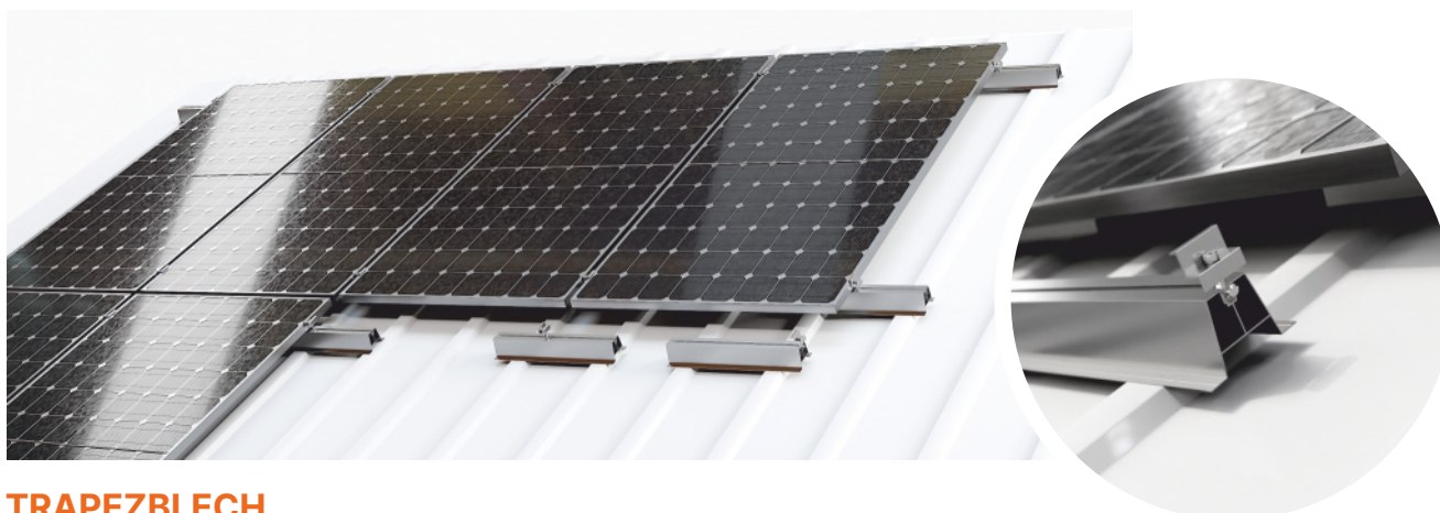
FALZBLECH
