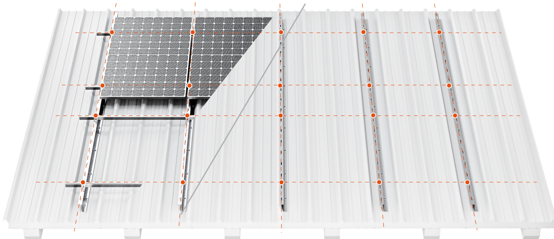
Profile „Z” layout
