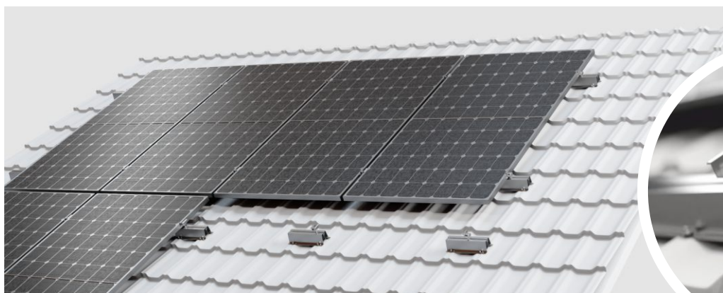
МЕТАЛОЧЕРЕПИЦЯ, КОНСТРУКЦІЯ НА МОСТАХ
