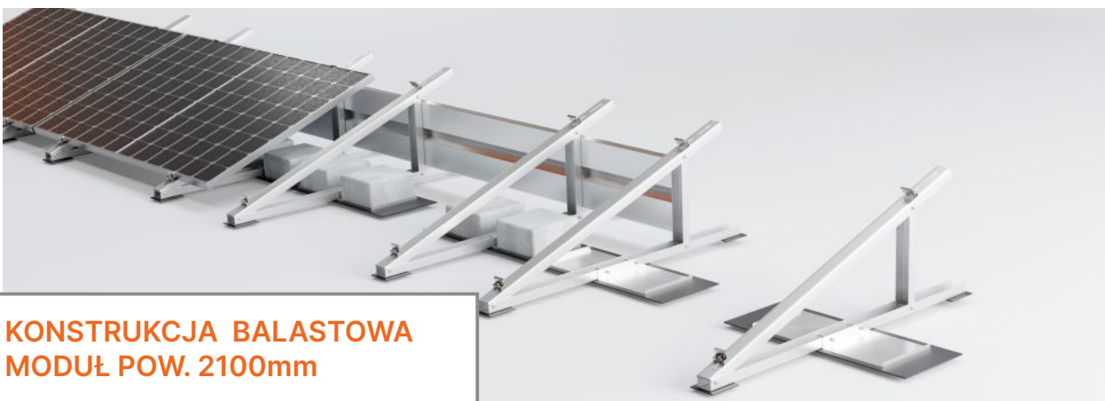
KONSTRUKCJA NA PŁYTĘ WARSTWOWĄ, POŁUDNIE 15/20° BIFACIAL
