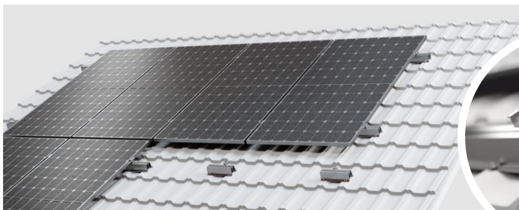
BLACHODACHÓWKA, KONSTRUKCJA NA MOSTEK
